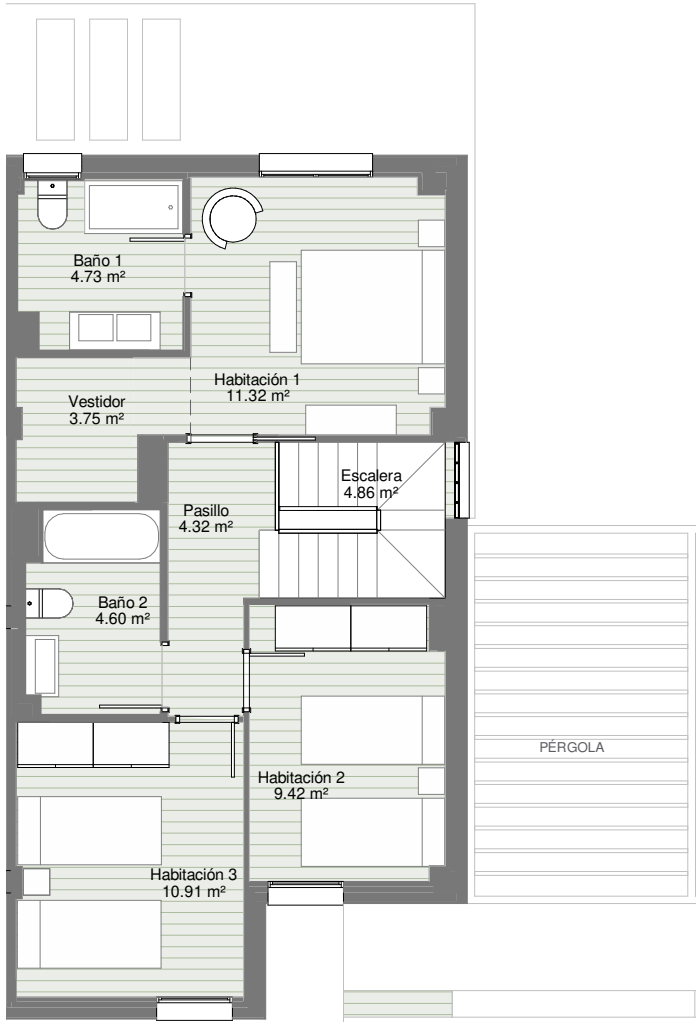
Planta Primera
