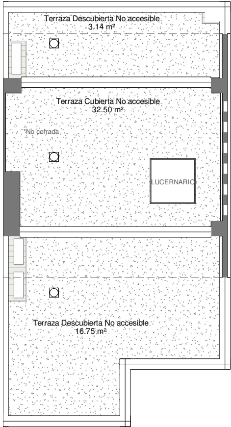
Planta Cubierta
