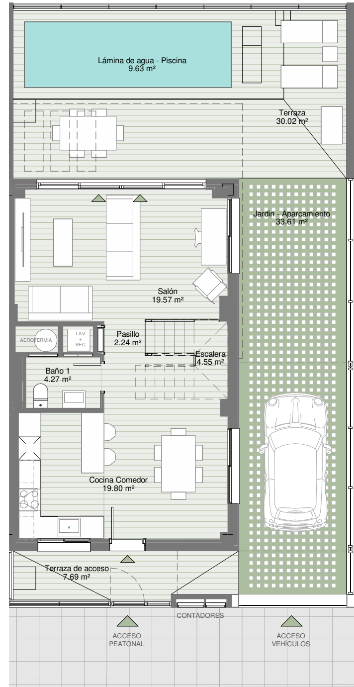
Planta Baja
